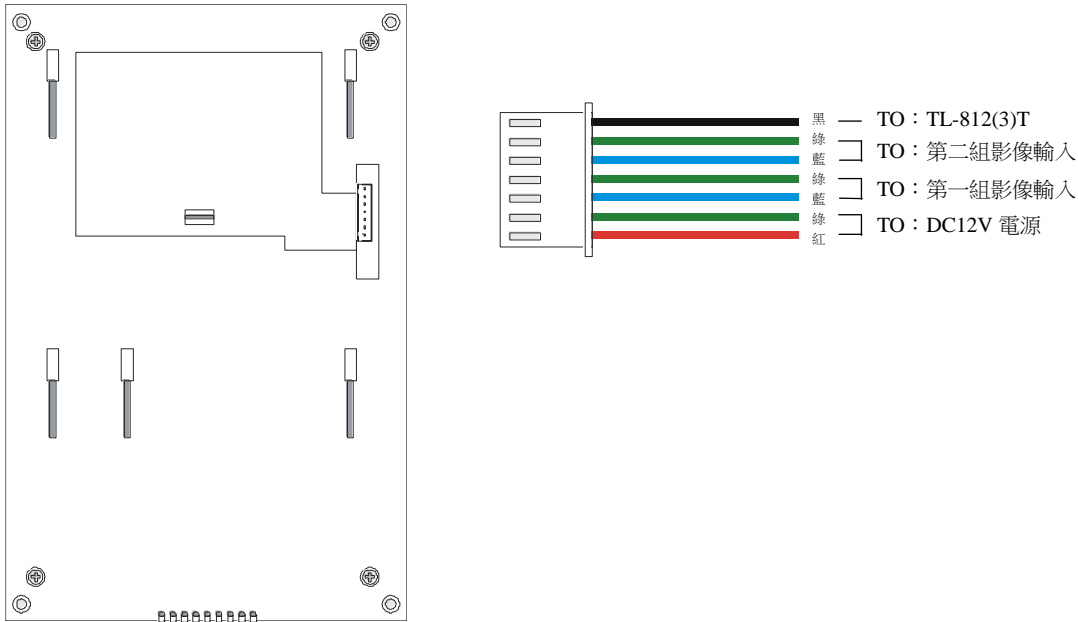
TL-212M/MC 背面接線圖
